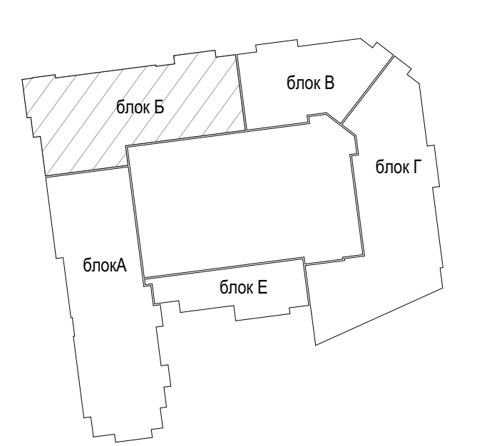
Разпределение на кота +2,88 /Блок Б/ М 1:50
